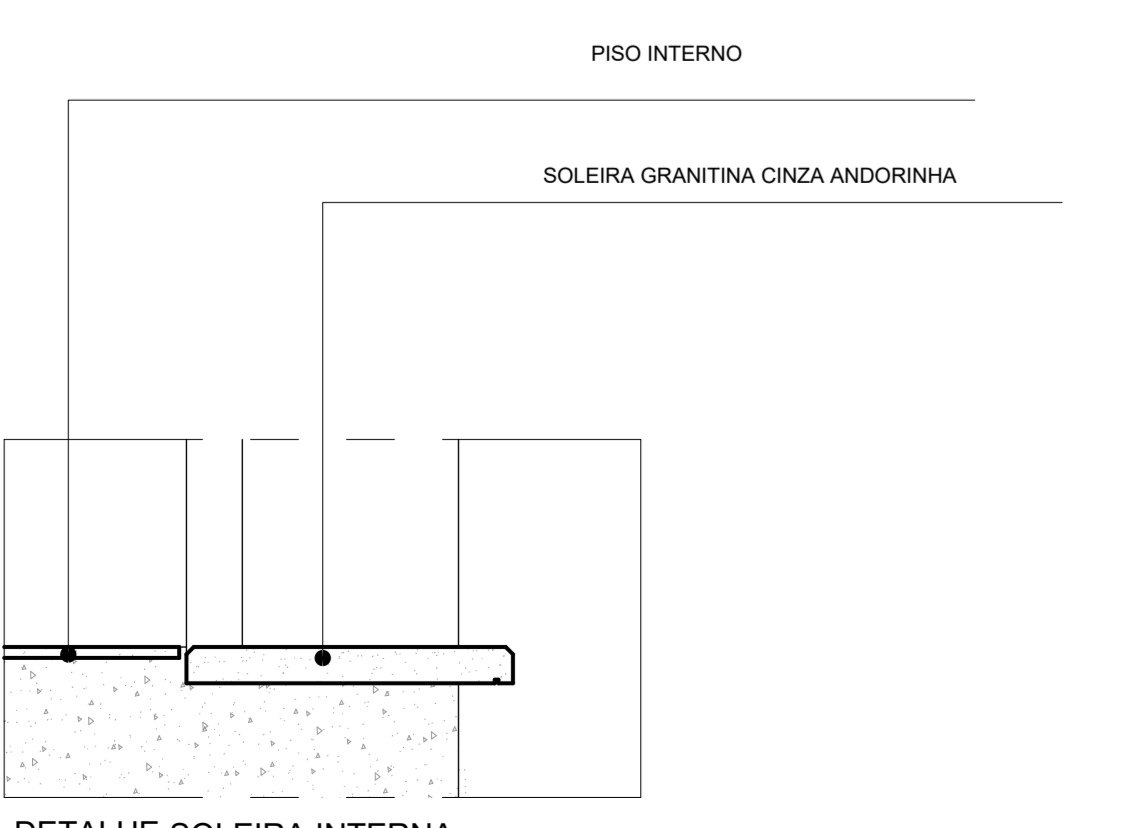
DETALHE SOLEIRA INTERNA ESCALA: 1/5
