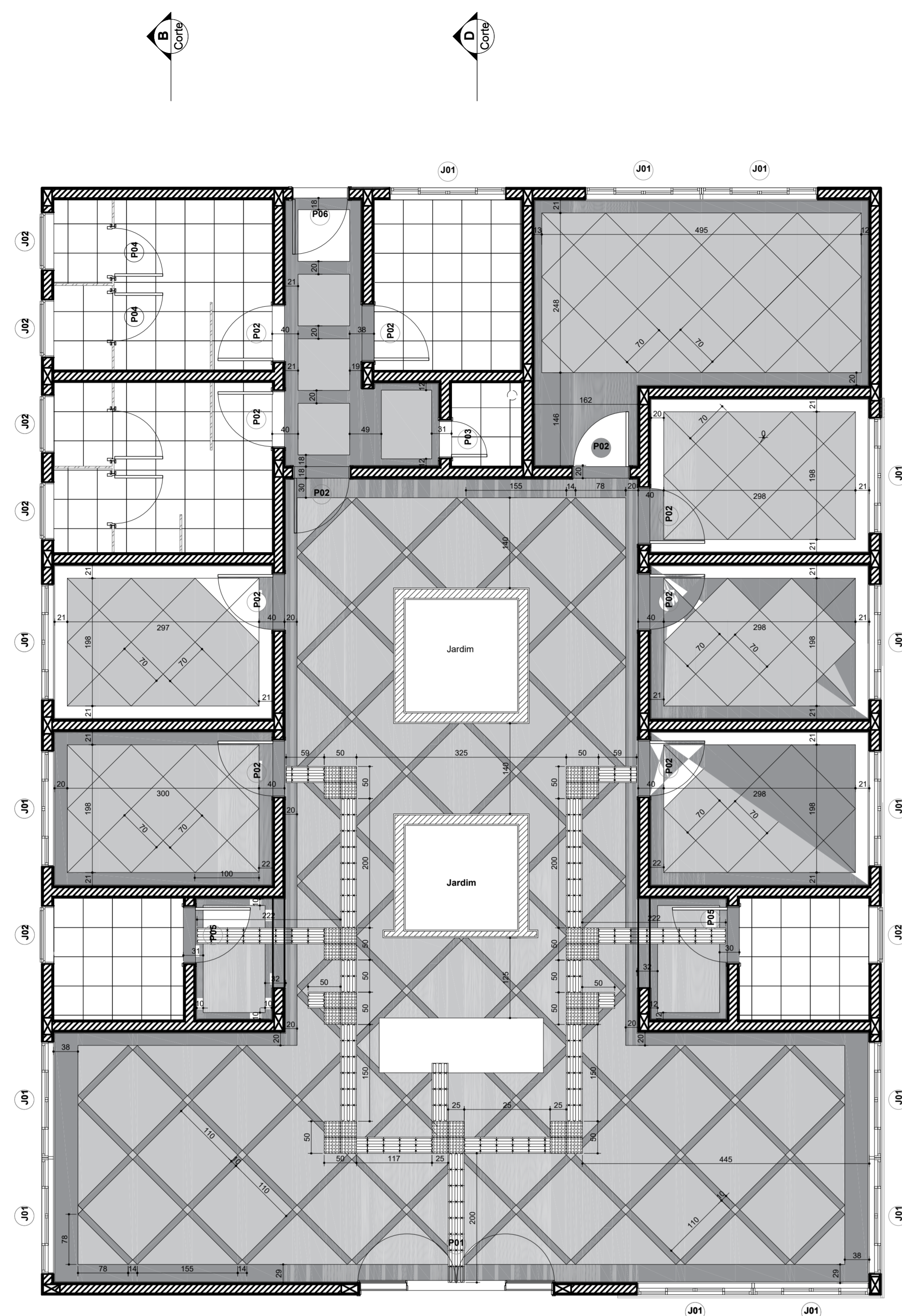
PLANTA PISO ESCALA 1:50
