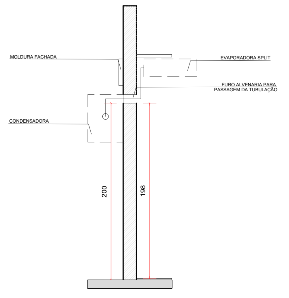
CORTE ESCALA 1:25
