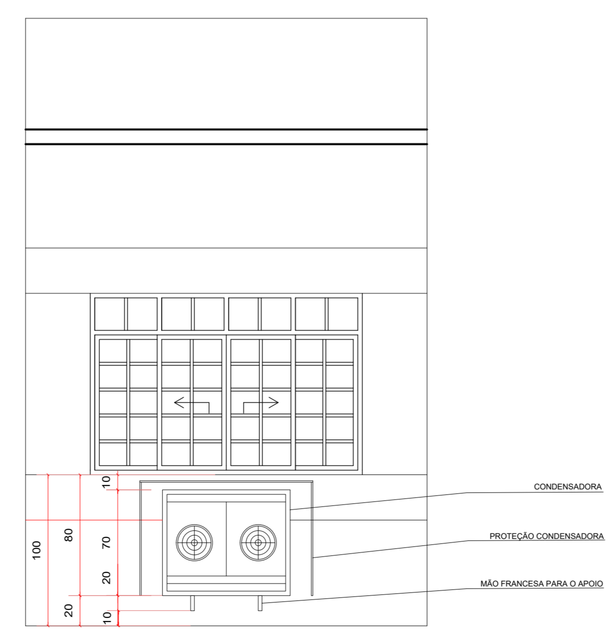
CORTE ESQUEMÁTICO ESCALA 1:25
