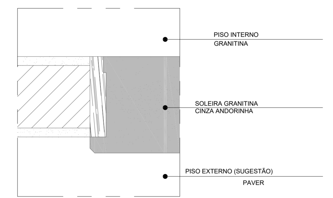
DETALHE SOLEIRA INTERNA ESCALA: 1/5
