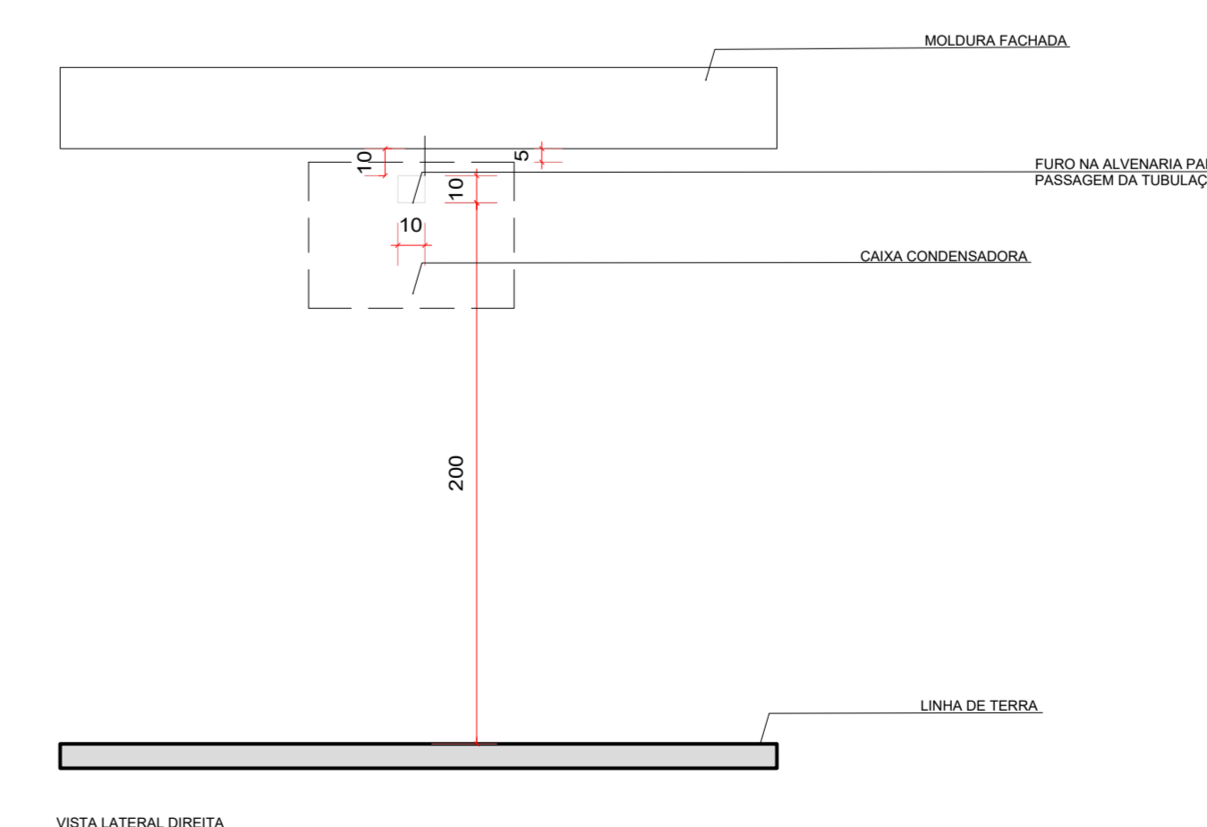
VISTA LATERAL DIREITA ESCALA 1:25
