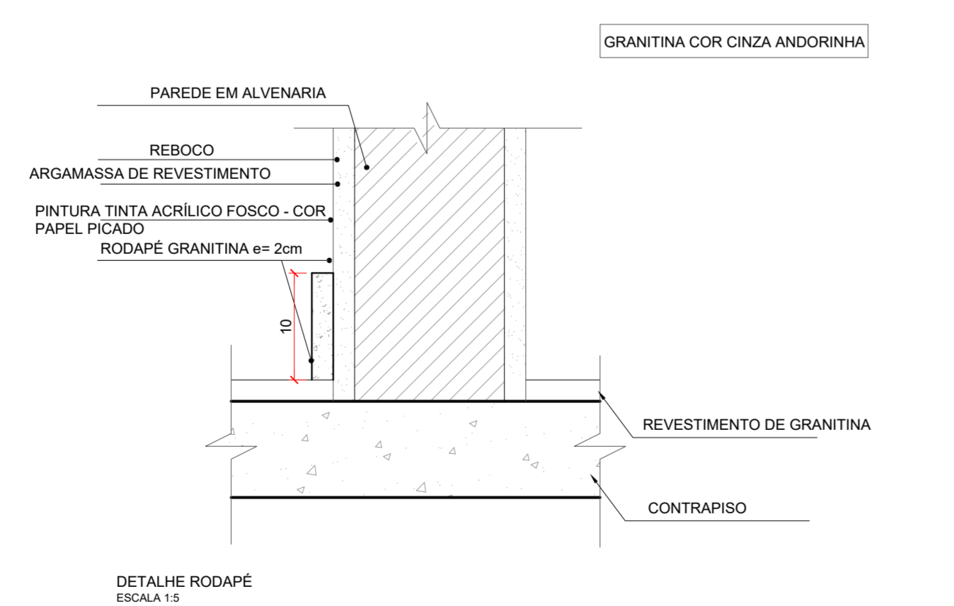
DETALHE PADRÃO PARA RODAPÉ DAS ÁREAS COM PISO EM GRANITINA (PAREDES EM ALVENARIA). ESCALA 1/5
