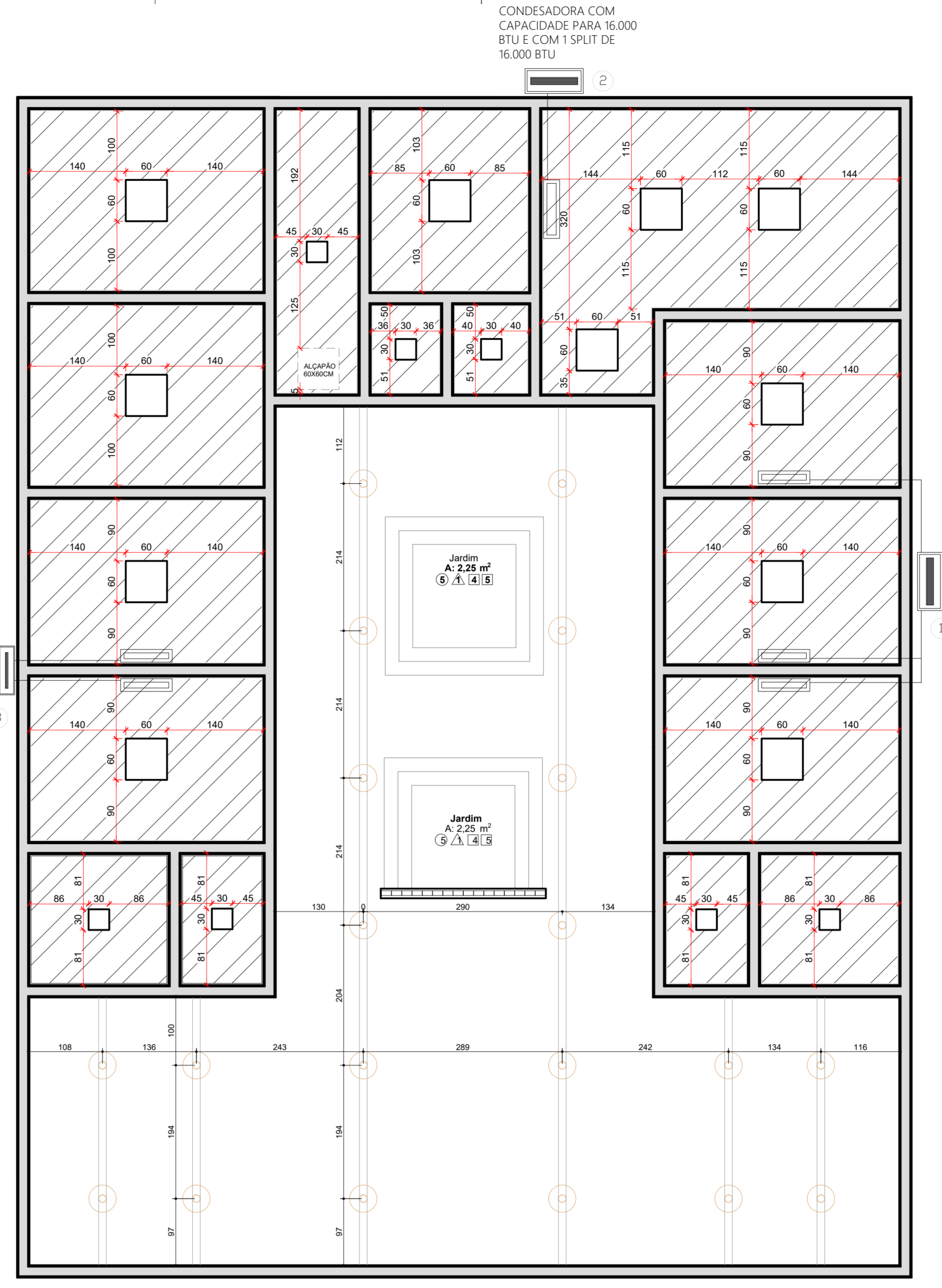
PLANTA FORRO/ELETRICA ESCALA 1:50
