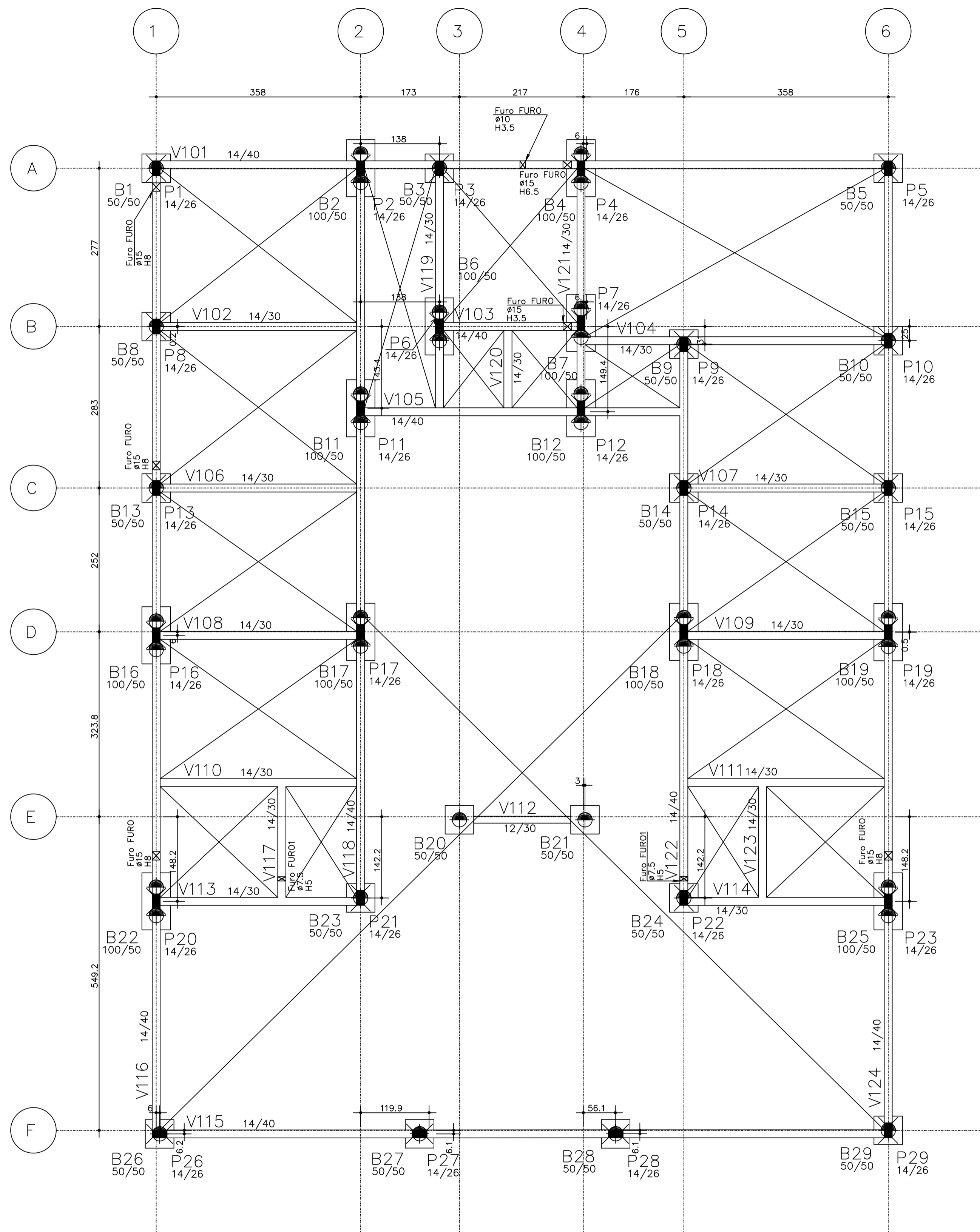
FORMAS FUNDAÇÃO – BLOCOS ESC 1/50
